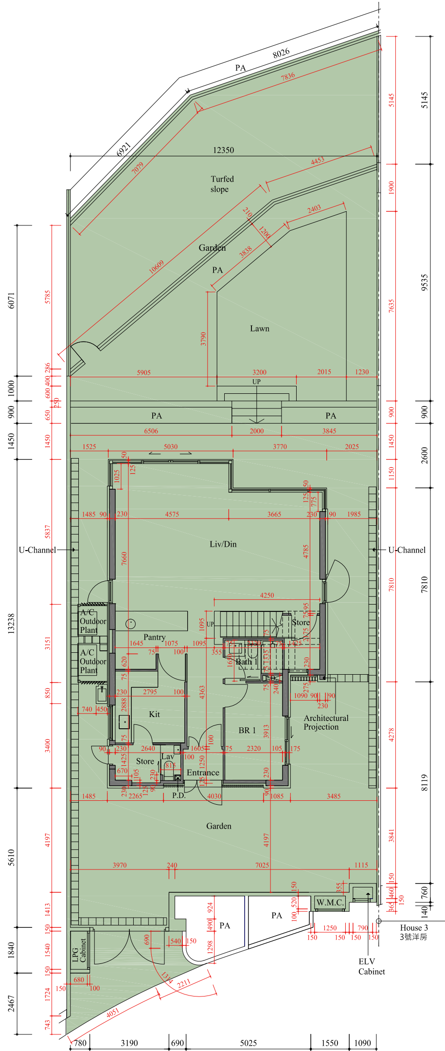
G/F FLOOR PLAN 地下樓面平面圖
